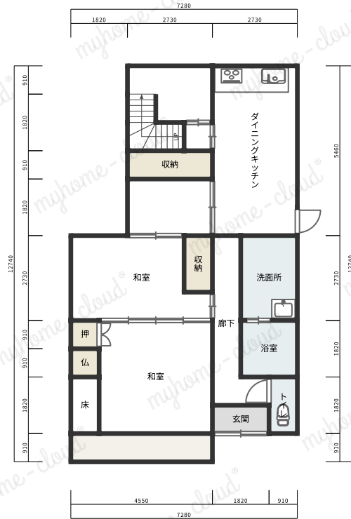
1階平面図
